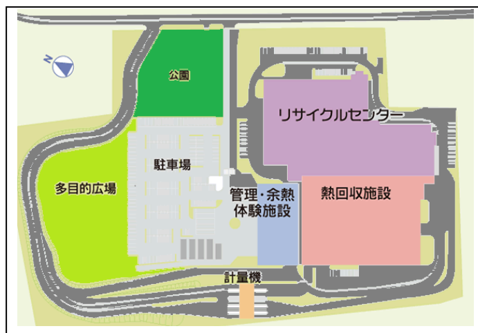
敷地配置図
